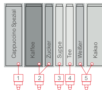
Variante 7501 B 7 Produktbehälter, 5 Mixereinheiten
